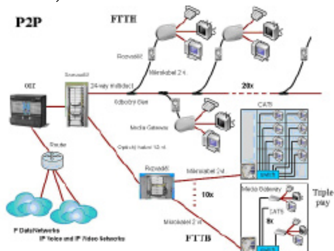
Obr. 2. Architektura pasivní optické přístupové sítě Point-To-Point
