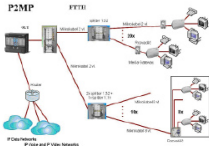
Obr. 3. Architektura pasivní optické přístupové sítě Point-To-Multipoint
